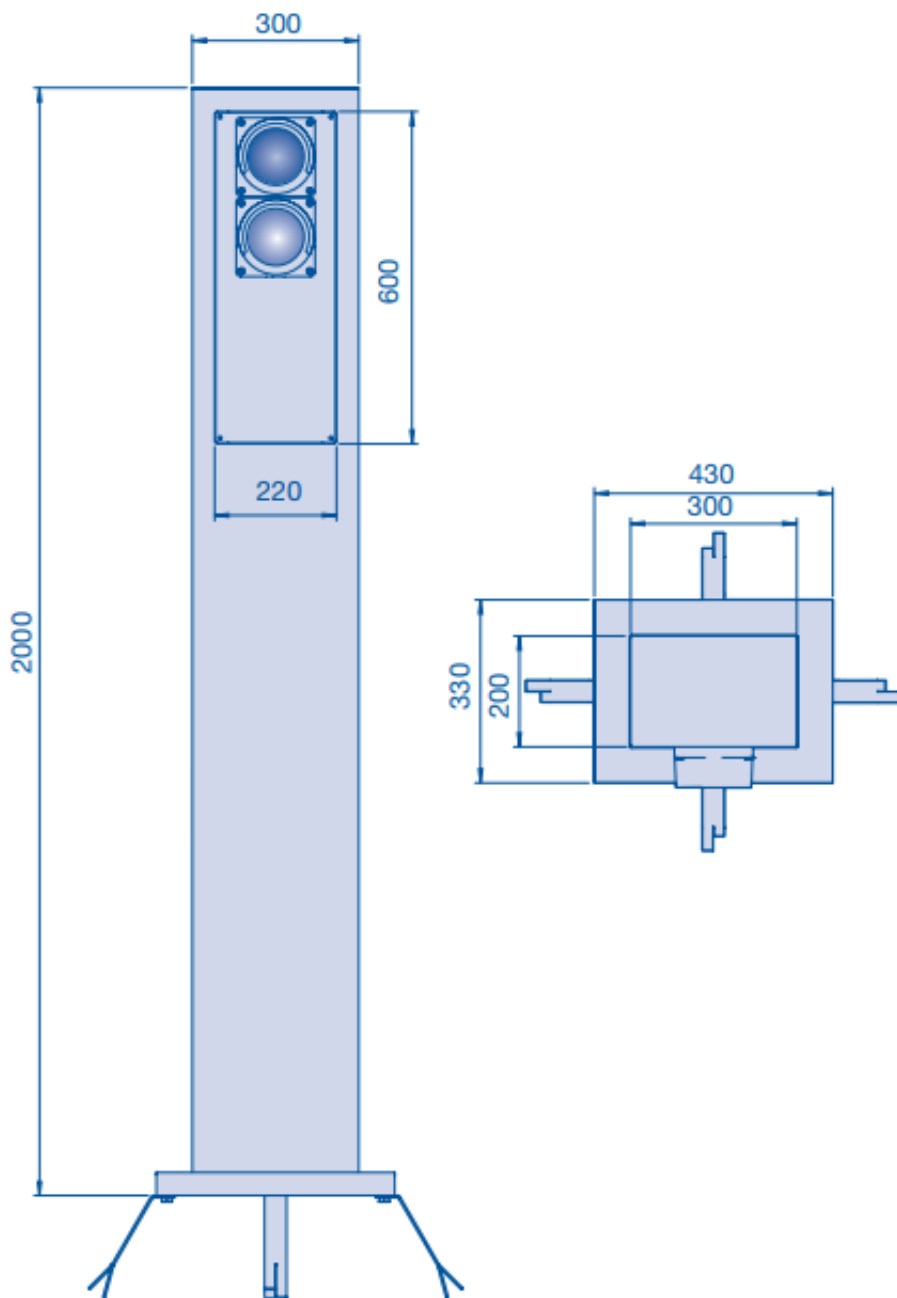
Rysunek z jednym wycięciem
