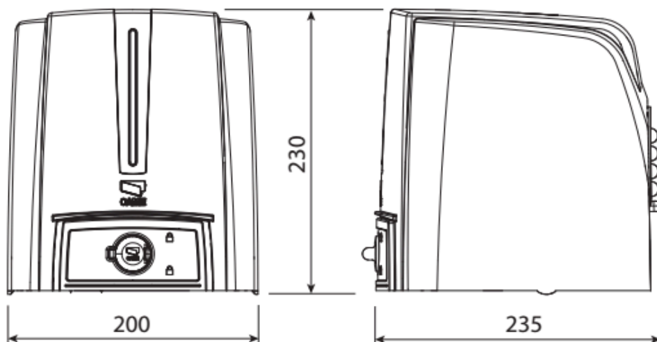
Montaż z ramieniem transmisyjnym przegubowym (standard)
